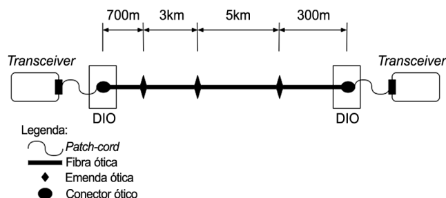
Figura 1: Visão sistêmica de enlace ótico.
